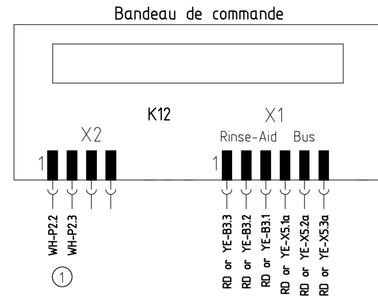
Capteur de manque de liquide de rinçage
