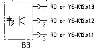
Capteur de manque de liquide de rinçage
